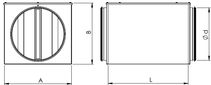
Ø 400-630
